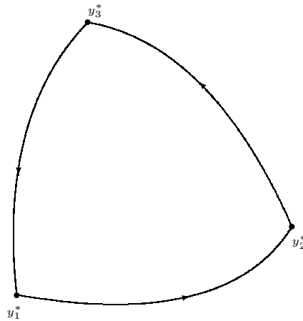
Estrutura homoclínica (1.4.1)
